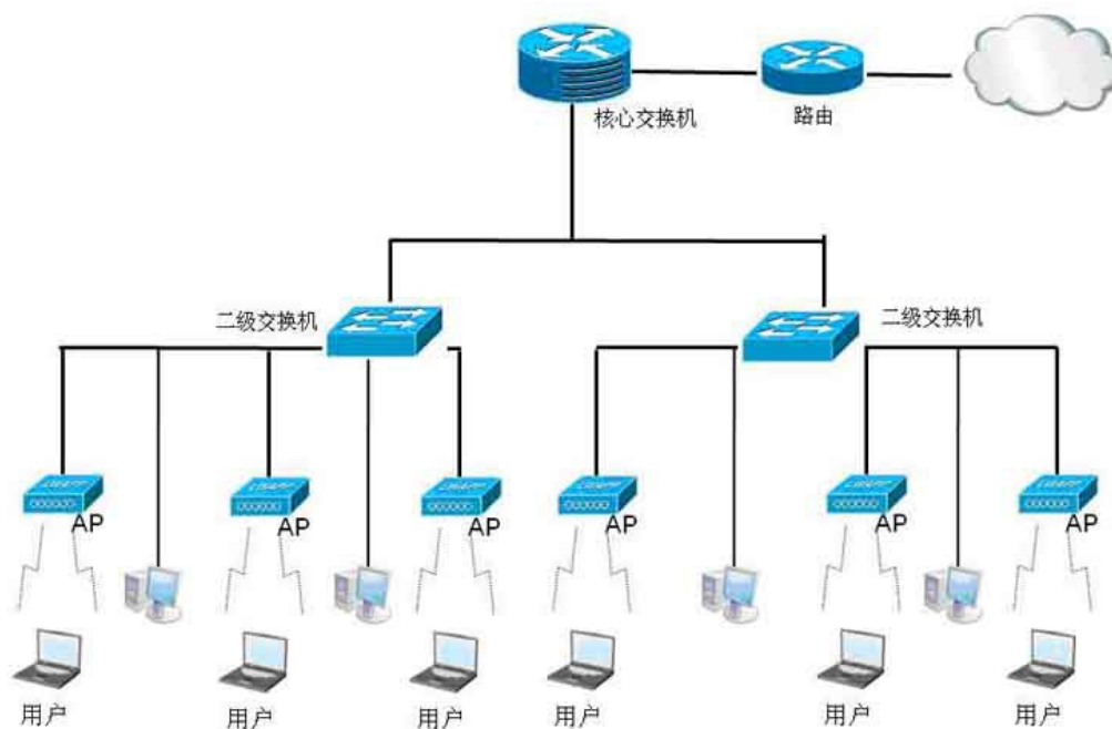
无线接入点拓扑图
